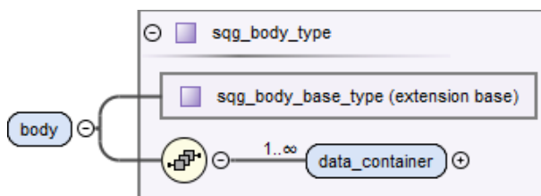
Abbildung 22: Aufbau des Elements body
