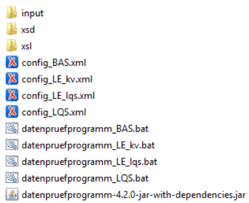
Abbildung 35: Verzeichnisstruktur eines DPP-Ordners
