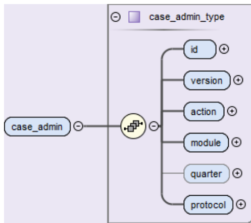
Abbildung 28: Aufbau des Elements case_admin
