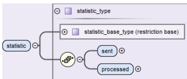
Abbildung 30: Aufbau des Elements statistic
