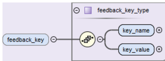
Abbildung 21: Aufbau des Elements feedback_key
