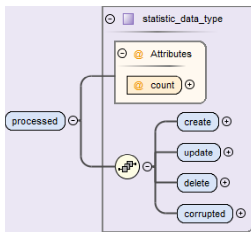
Abbildung 32: Aufbau des Elements processed
