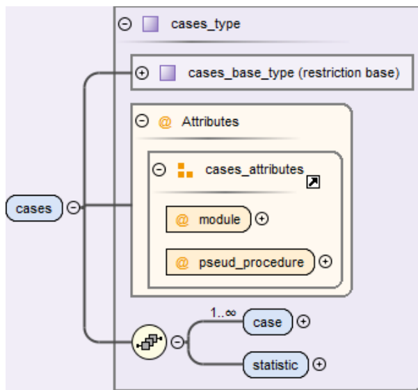
Abbildung 26: Aufbau des Elements cases
