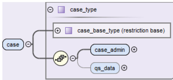
Abbildung 27: Aufbau des Elements case
