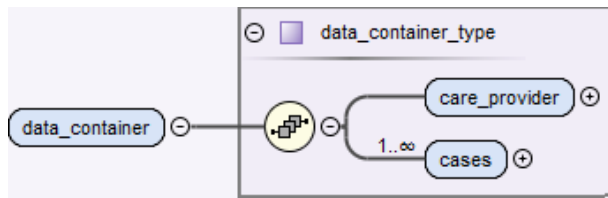
Abbildung 23: Aufbau des Elements body/data_container
