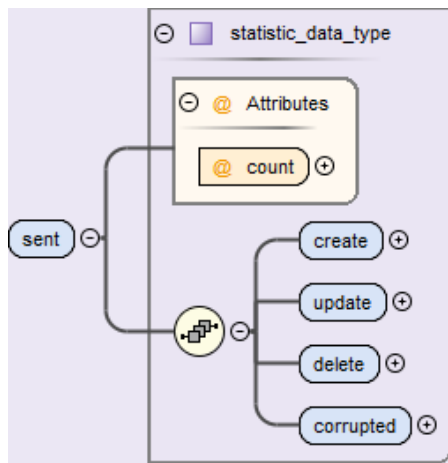
Abbildung 31: Aufbau des Elements sent
