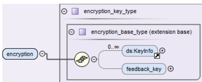
Abbildung 20: Aufbau und Attribute des Elements encryption (AP-selektiv/-kollektiv)
