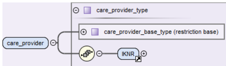
Abbildung 24: Aufbau des Elements care_provider – kollektiv-, selektivvertraglich
