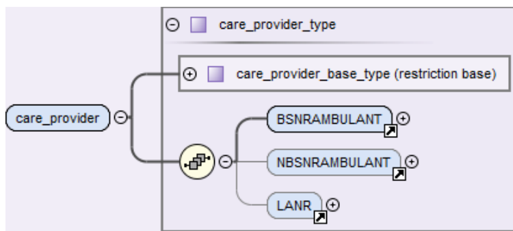
Abbildung 24: Aufbau des Elements care_provider – kollektiv-, selektivvertraglich
