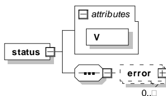
Abbildung 38: Aufbau und Kind-Elemente des Elements status
