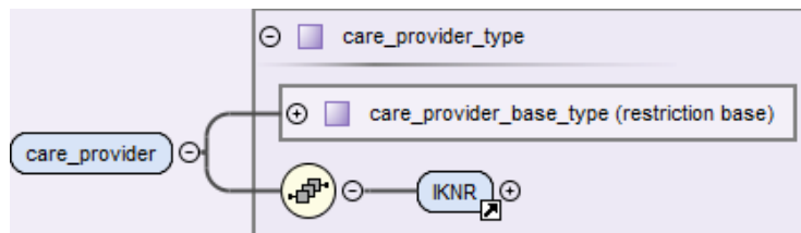
Abbildung 22: Aufbau des Elements care_provider – kollektiv-, selektivvertraglich
