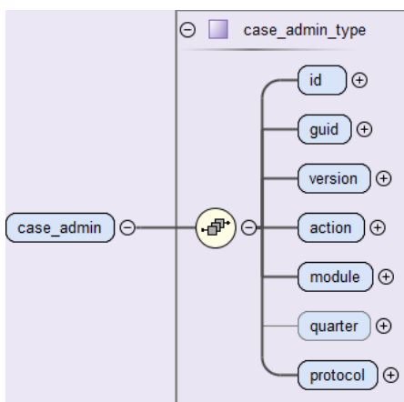
Abbildung 26: Aufbau des Elements case_admin Im Folgenden werden die einzelnen Kind-Elemente beschrieben.
