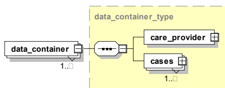
Abbildung 38: Aufbau des Elements body/data_container
