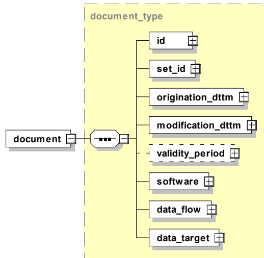
Abbildung 26: Aufbau des Elements document
