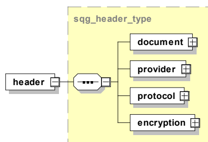
Abbildung 25: Aufbau des Elements header
