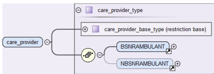
Abbildung 46: Aufbau des Elements care_provider – kollektiv-, selektivvertraglich
