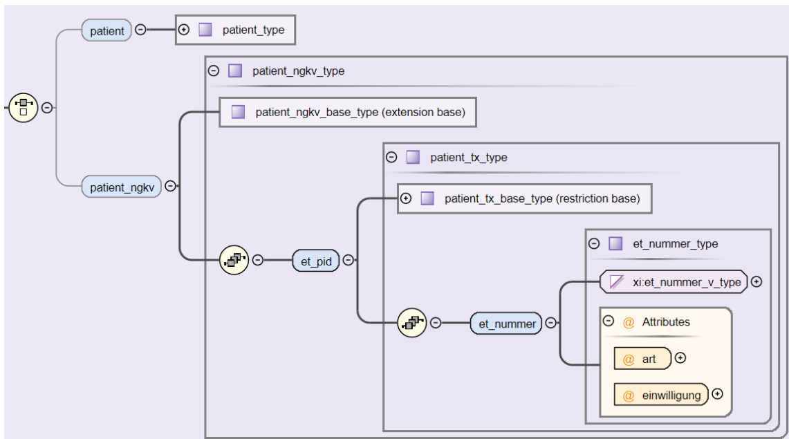
Abbildung 53: Aufbau des Elements patient_ngkv
