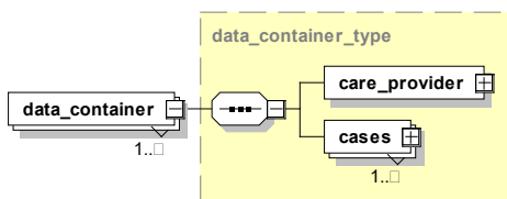
Abbildung 45: Aufbau des Elements body/data_container
