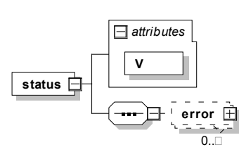
Abbildung 33: Aufbau und Kind-Elemente des Elements status
