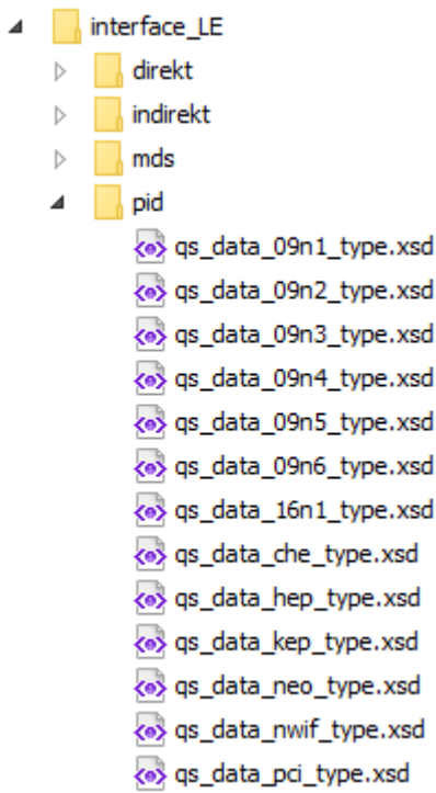
Abbildung 53: Ausprägungen des qs_data -Elements (Erfassungsmodule)
