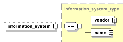
Abbildung 27: Aufbau des Elements information_system
