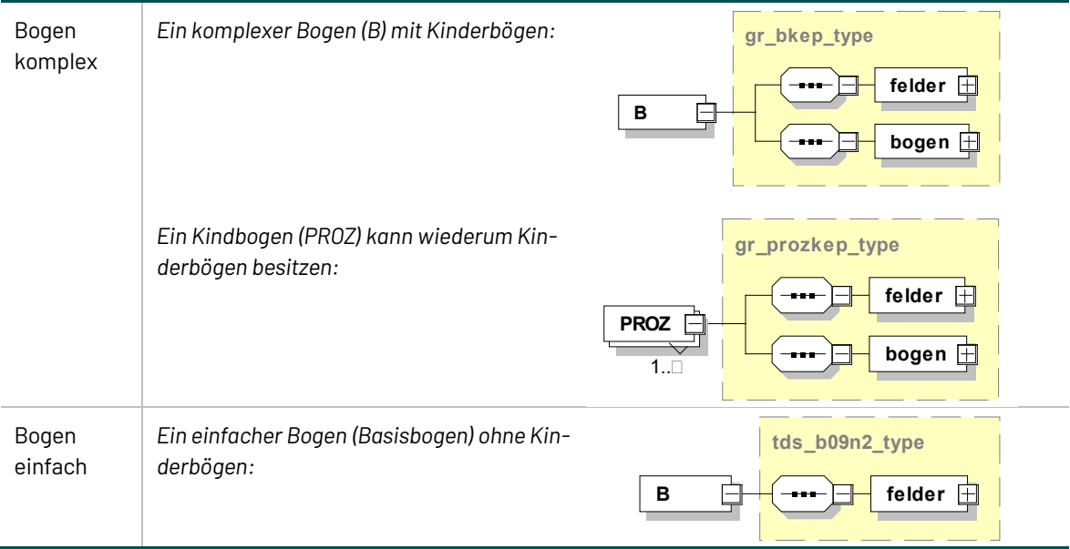
Abbildung 52: Diagramme „Bogen komplex“ und „Bogen einfach“
