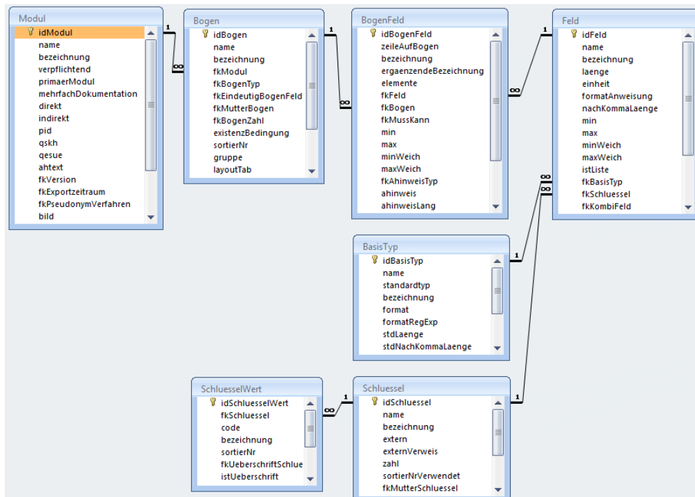
Abbildung 12: Tabellen und Relationen der Datenfeldbeschreibung (Beispiel Spezifikation 2017)
