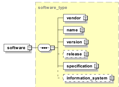
Abbildung 26: Aufbau des Elements software
