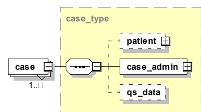
Abbildung 41: Aufbau des Elements case
